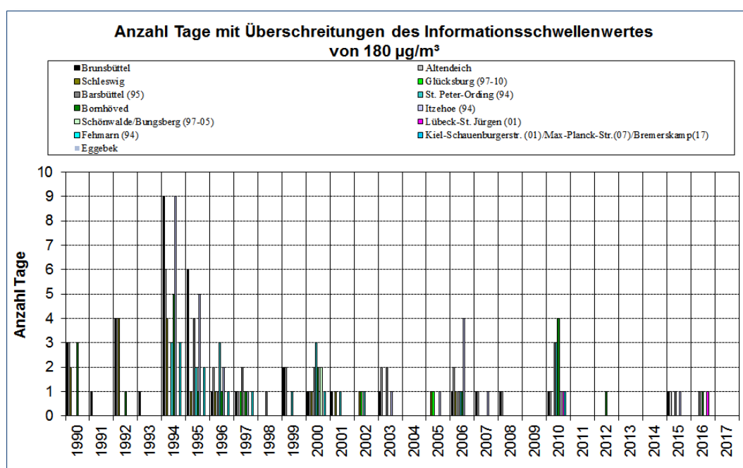
Abbildung 17: Anzahl der Tage mit Überschreitungen der Informationsschwelle, 1990 - 2017
