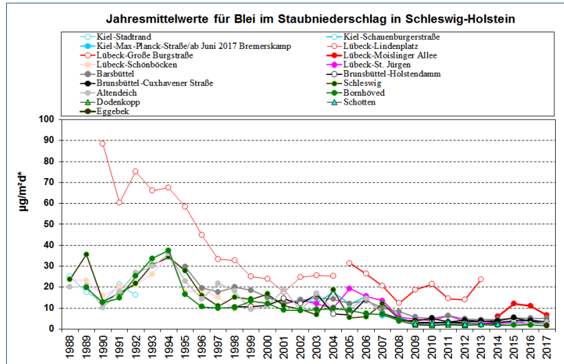
Abbildung 9: Jahresmittelwerte für Staubbiederschlag in Schleswig-Holstein, 1988 – 2017
