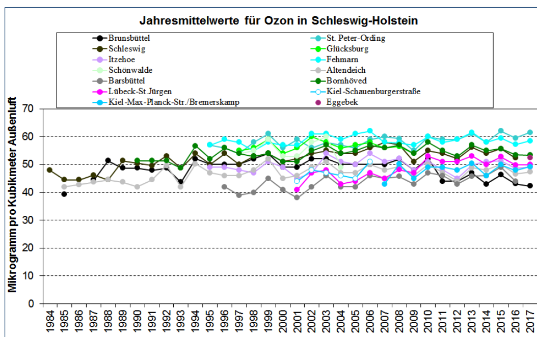
Abbildung 16: Jahresmittelwerte für Ozon in Schleswig-Holstein, 1984 – 2017
