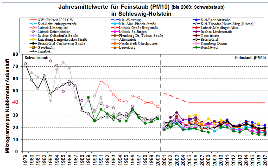
Abbildung 2: Jahresmittelwerte für Schwebstaub und Feinstaub (PM10) in Schleswig-Holstein, 1979 – 2017
