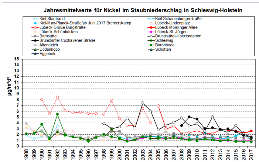
Abbildung 12: Jahresmittelwerte für Nickel im Staubniederschlag in Schleswig-Holstein, 1988 - 2017
