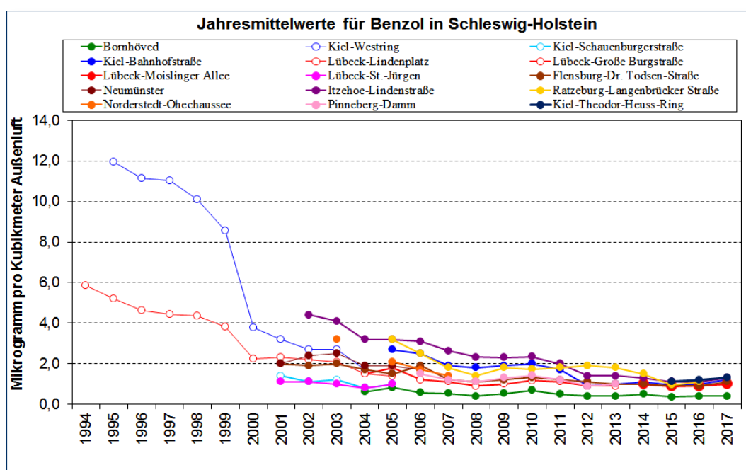
Abbildung 15: Jahresmittelwerte für Benzol in Schleswig-Holstein, 1994 – 2017
