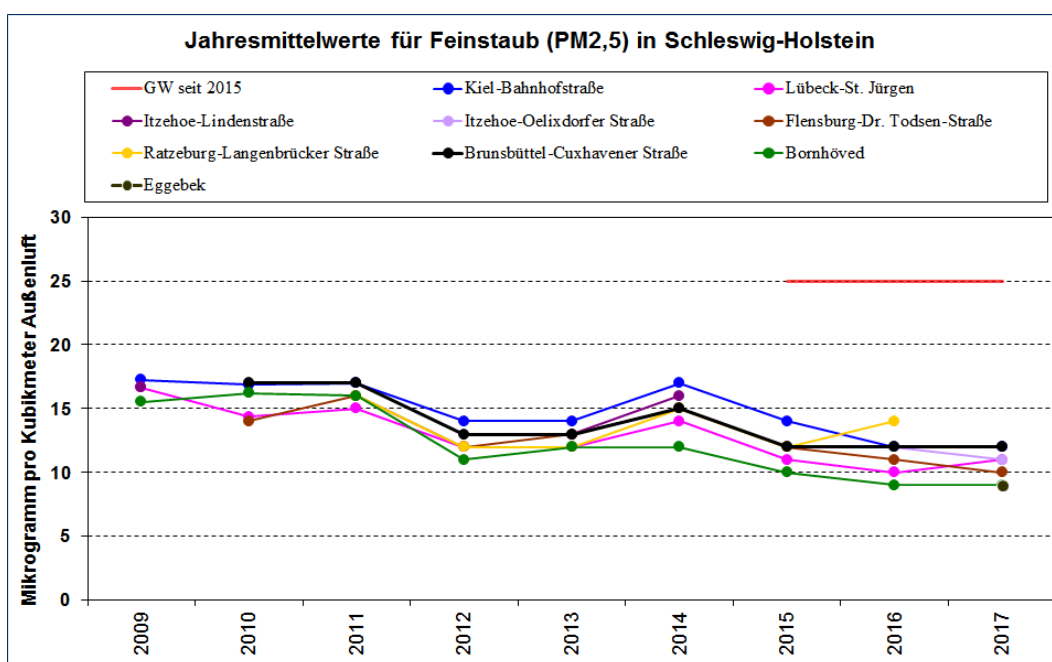
Abbildung 3: Jahresmittelwerte für Feinstaub (PM 2,5 ) in Schleswig-Holstein, 1979 – 2017
