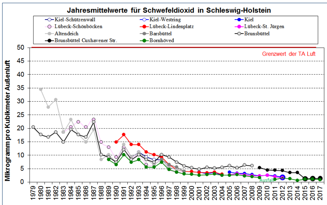
Abbildung 1: Jahresmittelwerte für Schwefeldioxid in Schleswig-Holstein, 1979 – 2017
