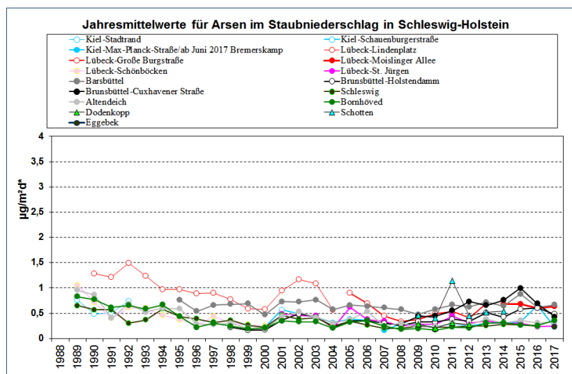
Abbildung 13: Jahresmittelwerte für Arsen im Staubniederschlag in Schleswig-Holstein, 1989 - 2017
