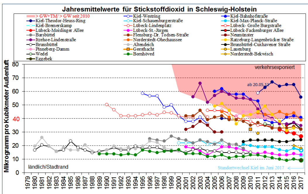
Abbildung 14: Jahresmittelwerte für Stickstoffdioxid in Schleswig-Holstein, 1980 – 2017
