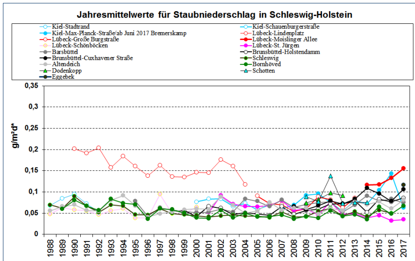
Abbildung 9: Jahresmittelwerte für Staubbiederschlag in Schleswig-Holstein, 1988 – 2017
