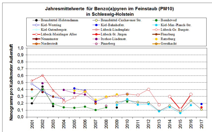
Abbildung 8: Jahresmittelwerte für Benzo(a)pyren im Feinstaub (PM10) in Schleswig-Holstein, 2001 - 2017
