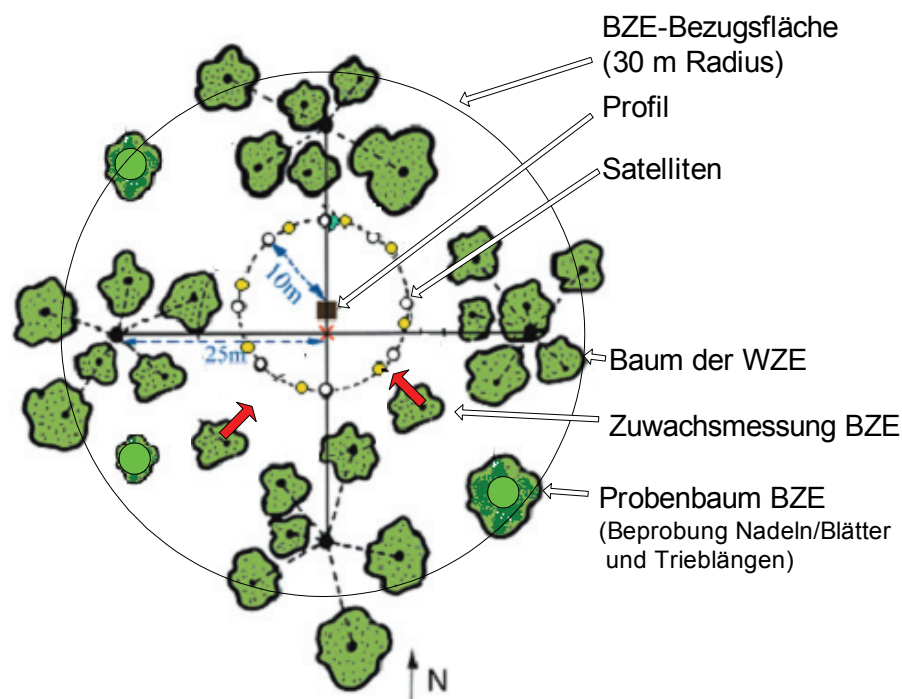
Abbildung 8: Schematische Darstellung des Aufnahmeverfahrens der BZE II
